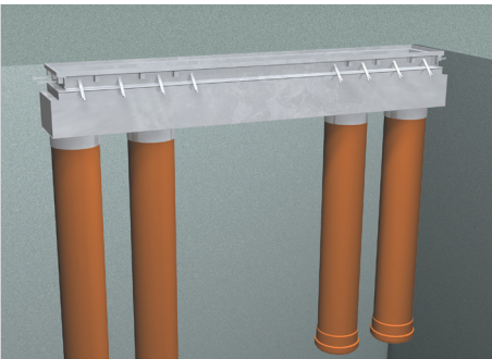
Hosenkassette Universal Stahl verzinkt 1500/2530 mm 275110
