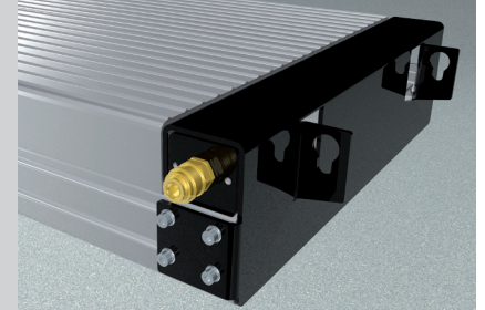
Druckluftversorgung 102407
