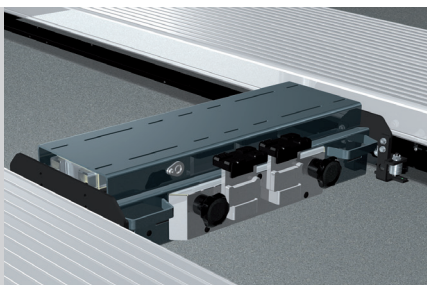
Achsheber 2600 kg pneumatisch, ohne Laufschiene
